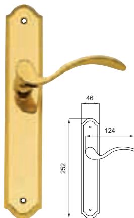
564 Maniglia Paperino H su placca Classic Paperino H door handle on Classic plate
