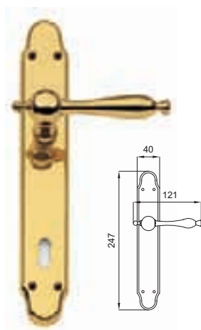
380 Maniglia su placca Door handle on plate
