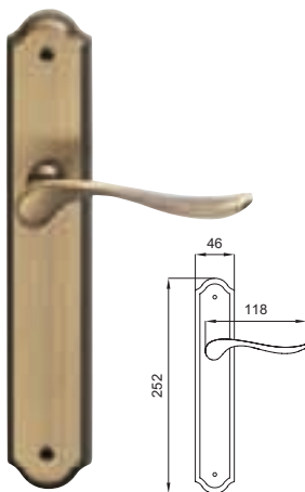
561 Maniglia su placca Classic Door handle on Classic plate
