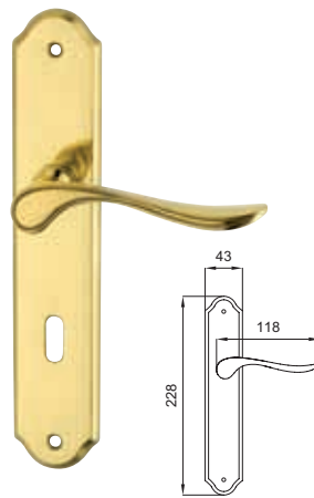
350/V Maniglia su placca Vienna Door handle on Vienna plate
