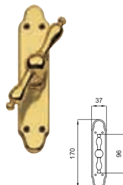
382 Cremonese con meccanismo Window handle with mechanism
