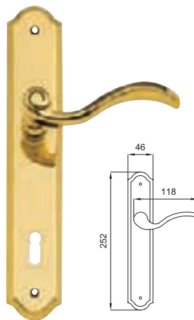
562 Maniglia su placca Classic Door handle on Classic plate
