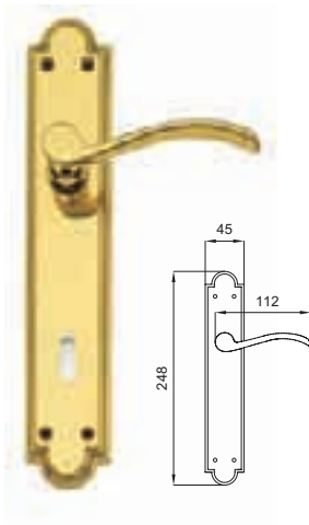
477 Maniglia su placca Door handle on plate
