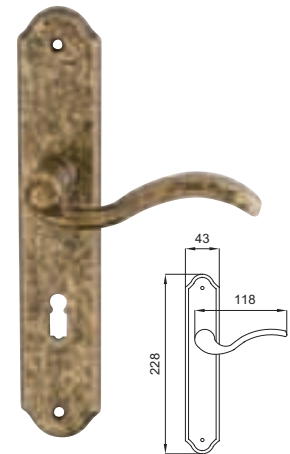
464/V Maniglia su placca Vienna Door handle on Vienna plate
