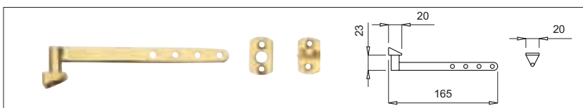
2253 Fermafinestre - Fermapersiane "Block" con 4 posizioni di bloccaggio. Basi girevoli, adattabili a finestre e persiane. Lunghezza 165 mm Casement and shutter stay with 4 blocking positions. Turnable basis, suitable to windows and shutters, 165 mm length
