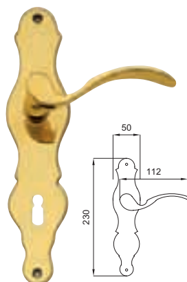
449/H Maniglia Paperino H su placca Paperino H door handle on plate
