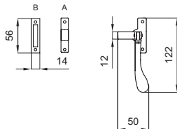
2262 Maniglia blocco reversibile Reversible mortice casement fastener
