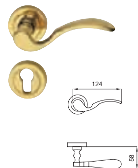
447 Maniglia Paperino H su rosetta e bocchetta ottone 50 mm Paperino H door handle on brass rose and escutcheon 50 mm
