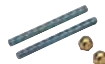
ASTD#06070ZI Set 2 tronconi M6 x 70mm zincati + 2 dadi ottone ciechi M6 Set of 2 zink M6 x 70mm bolts + 2 M6 blind screw nuts
