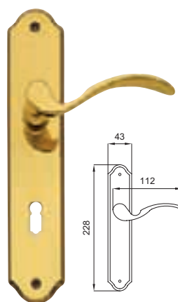
451/H Maniglia Paperino H su placca Vienna Paperino H door handle on Vienna plate
