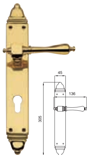
472 Maniglia su placca Door handle on plate
